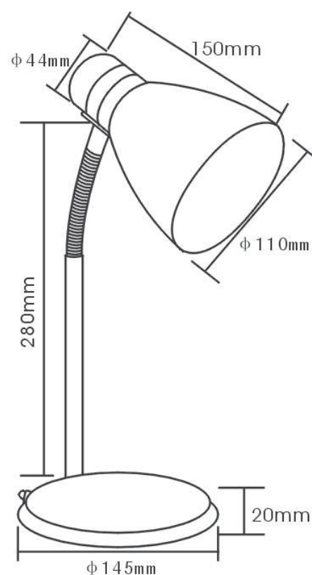
GRÁFICO CON DIMENSIONES (en mm)
